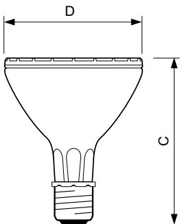
CDM-R 70W/830 E27 PAR30L 30D
