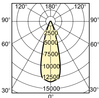
CDM-R 70W /830 PAR30L 30D
